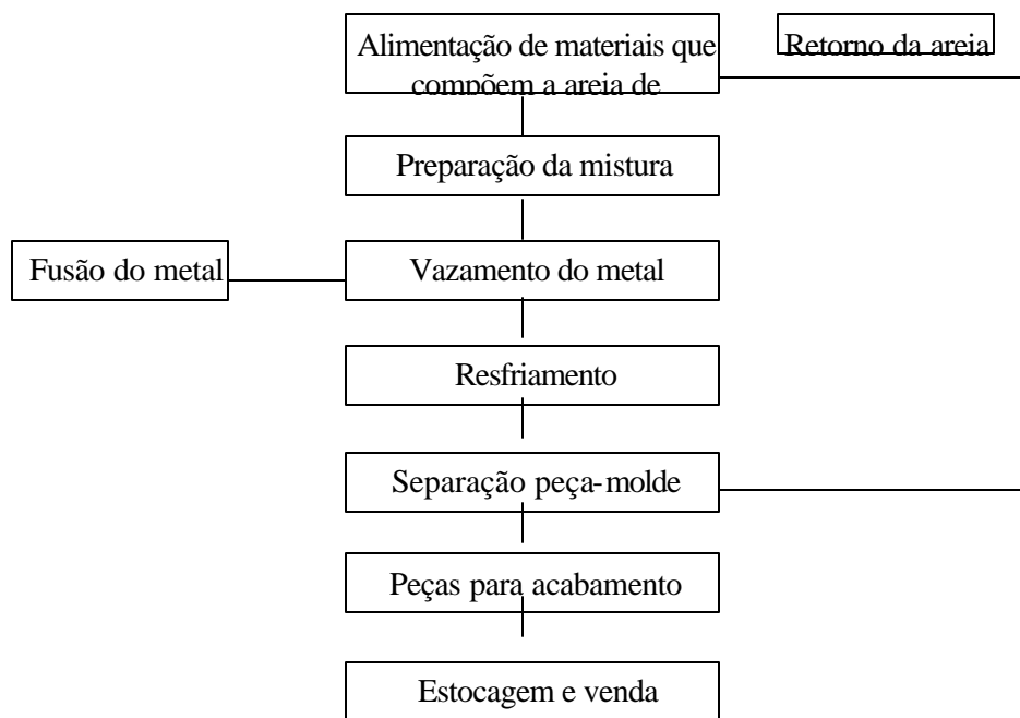
Figura 02 - Fluxograma de um processo usual de fundição.
